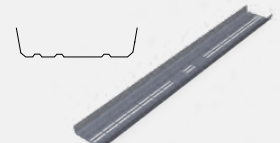
TRI-FLAT Easyspeed Ballastwanne Kies 2025 / 2225 / 2475
