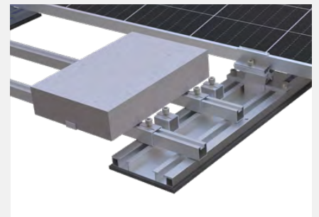
Beispiel: Verwendung der Ballastclips bei kurzem Reihenabstand.
