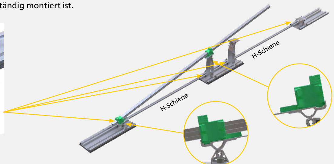
Fixierung der H-Schienen mittels M8 x12 Schraube
