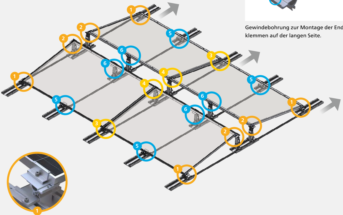
Endklemme am Modulfeldrand
