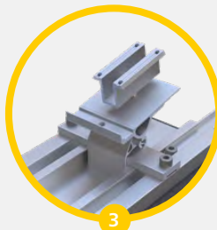
Mittelklemme zwischen zwei Modulen
