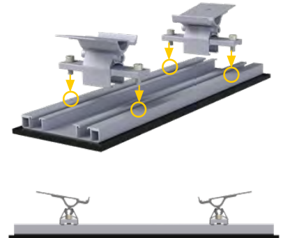
Montage der Stütze klein – langer Abstand
