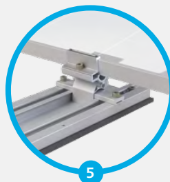
Endklemme als Verstärkung an Mittelmodule
