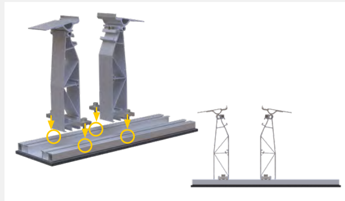
Montage der Stütze groß – kurzer Abstand
