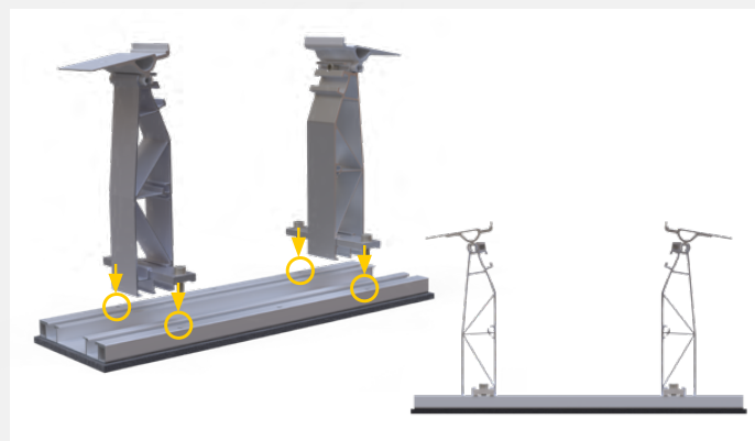
Montage der Stütze groß – langer Abstand
